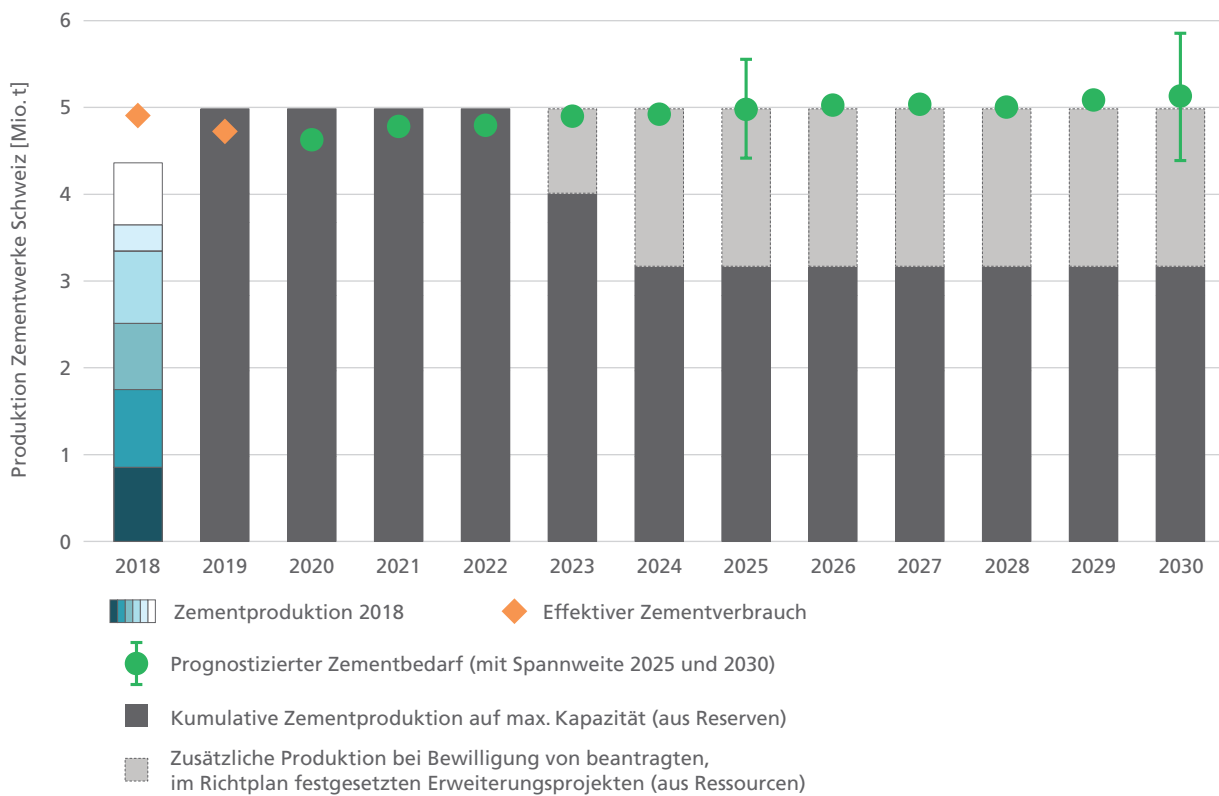
Fig. 18: Prognostizierte, kumulative Zementproduktion der sechs Zementwerke auf Grundlage der aktuellen Abbaubewilligungen (Reserven) und unter Annahme einer Produktion auf maximaler Kapazität, effektiver Zementverbrauch (Stand Ende 2019) und prognostizierter Bedarf bis 2030 mit der Spannweite der Szenarien in 2025 und 2030 (s. Kap. 3). Die hellen Balken zeigen den Fall, in dem alle im Richtplan festgesetzten Erweiterungsprojekte bis 2023 bewilligt und somit alle vorhandenen Ressourcen in Reserven umgewandelt würden. Die Farben der Säule für das Jahr 2018 entsprechen der tatsächlichen Produktion der einzelnen Zementwerke. Quelle: swisstopo, Erhebung Q1/2019, basierend auf Angaben der einzelnen Werke und Kantone.
