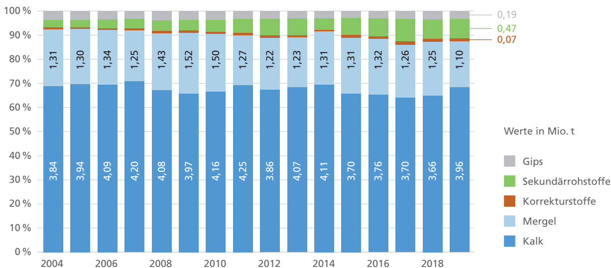
Fig. 17: Verbrauch von Zementrohstoffen 2004–2019 [6]. Siehe Kapitel 5.3 für eine Zusammenstellung der eingesetzten Sekundärrohstoffe.
